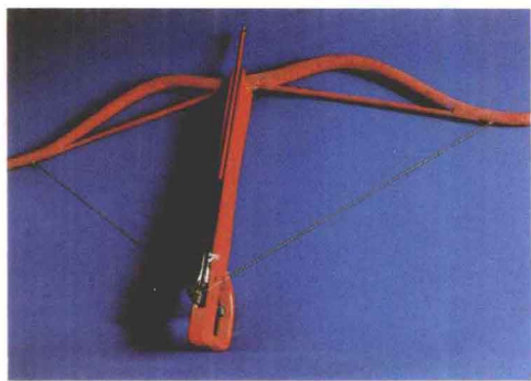
秦 青铜弩修复完整图
