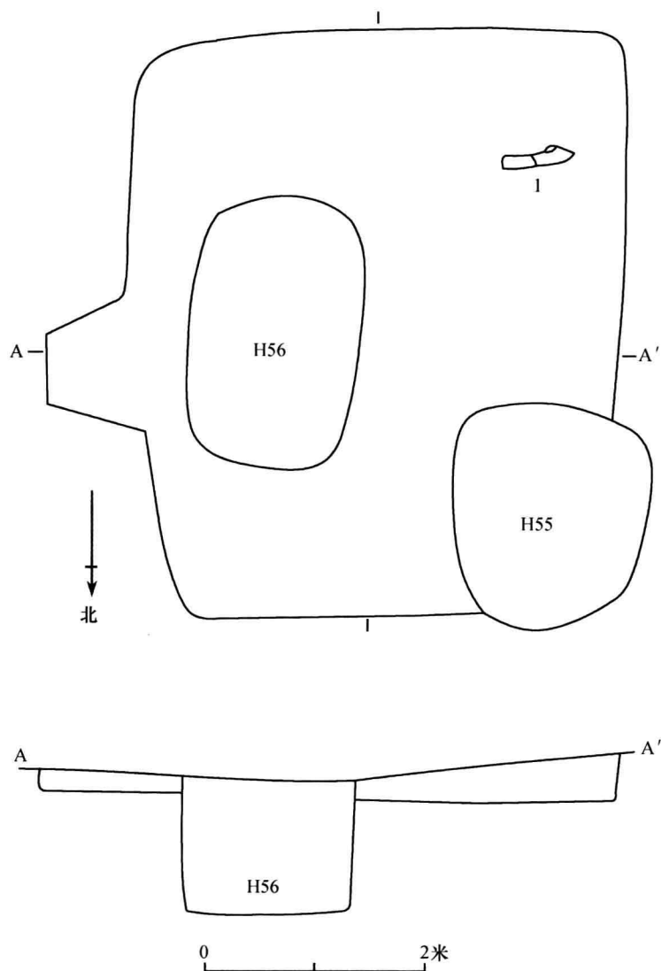
图 8 BF42 平、剖面图
