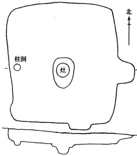
图 6 西梁 F107 平、剖面图
