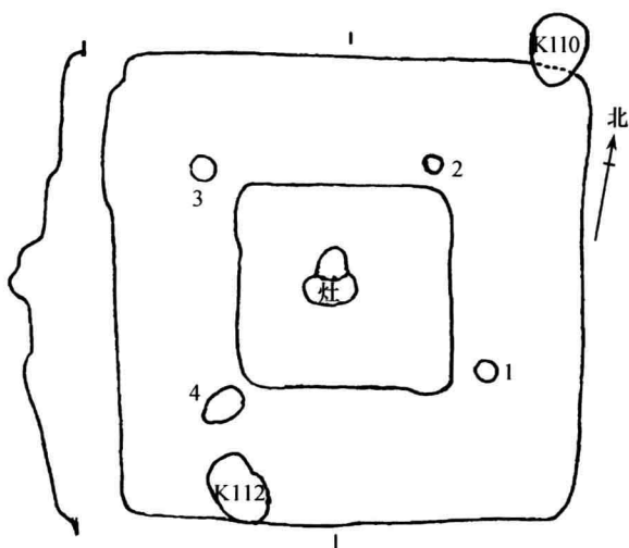
图4 西梁 F110 平、剖面图 1~4. 柱洞 K110、K112 为房址浅坑
