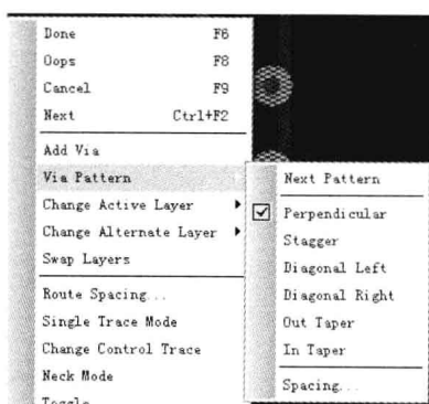
图 1-4-7 群组布线导通孔类型选择
