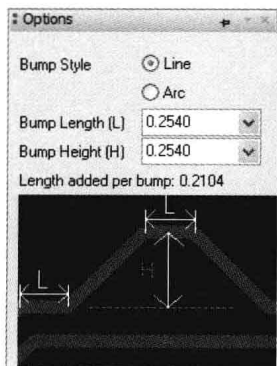
图 1-4-5 “Options” 选项卡
