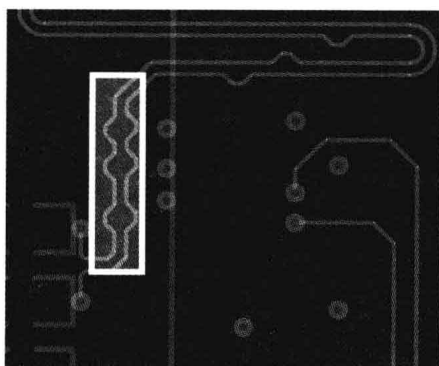
图 1-4-6 相位调整效果
