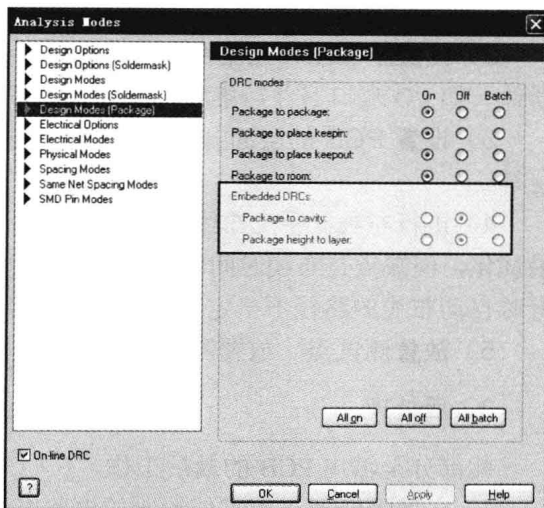
图 1-4-2 Embedded DRCs 设置界面
