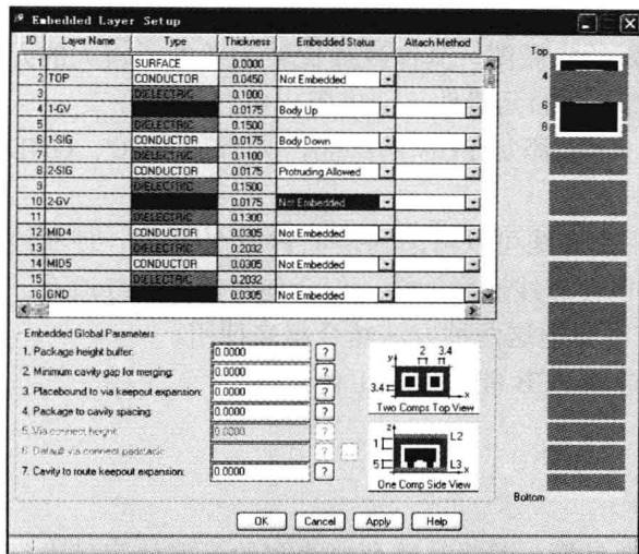
图 1-4-1 嵌入层设置界面
