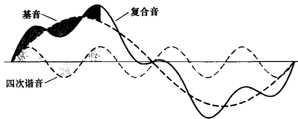
图 1-3 复合音被分解成基音和四次谐音的示意图
