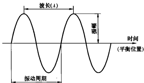
图 1-2 质点的位移幅度与时间变化的关系
