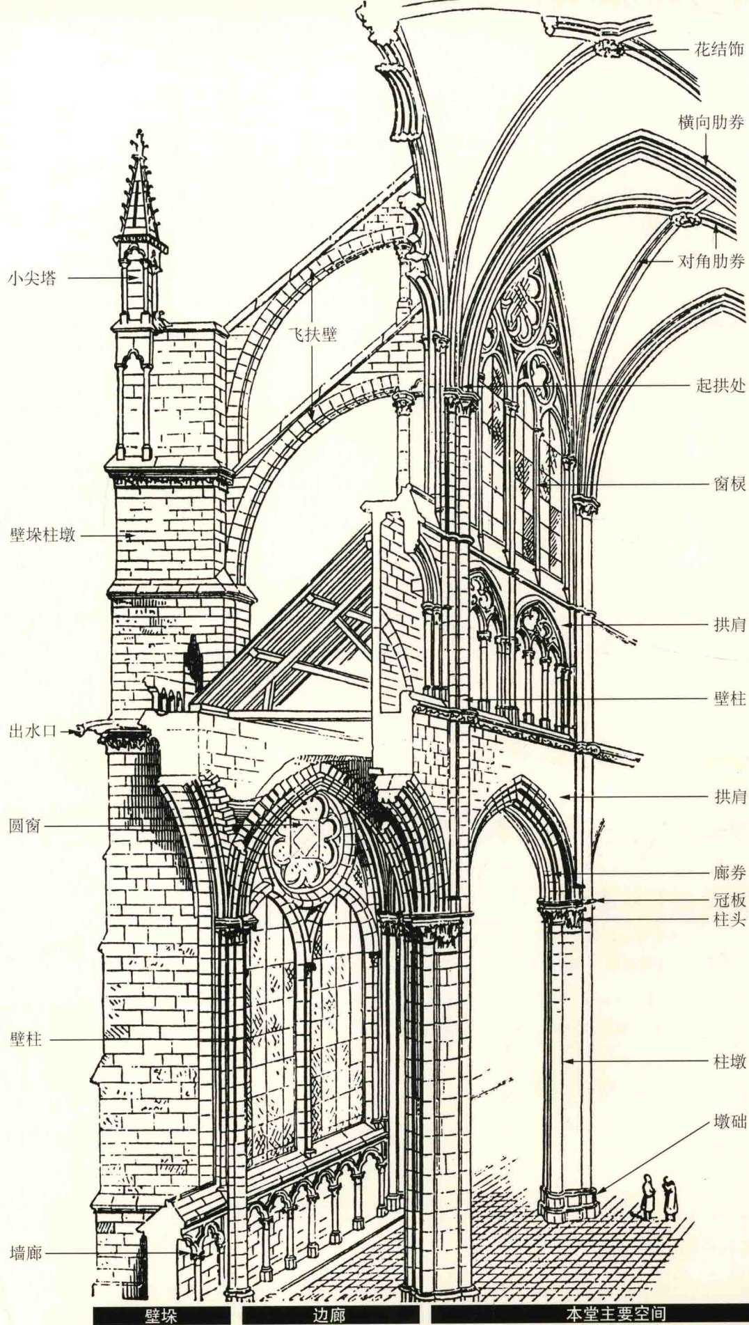
典型哥特教堂构造及各部名称图 (据 Eugène E. Viollet-le-Duc, 以亚眠大教堂为例)
