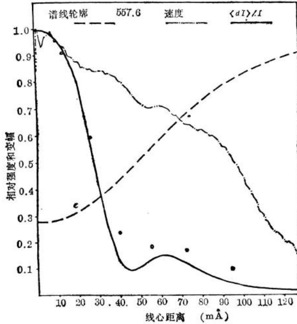
图 3 \lambda 5577 的轮廓和振荡
