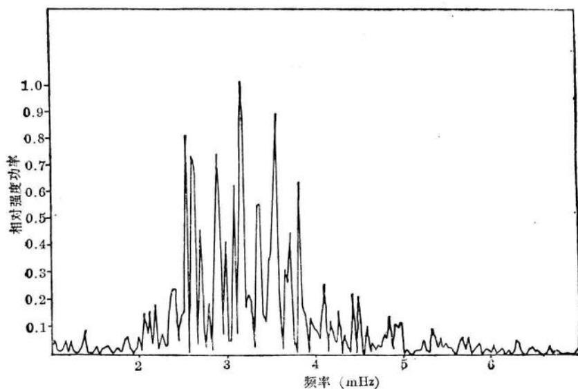
图2 线心强度变化的功率谱
