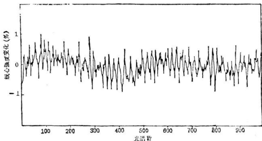
图1 FeI \lambda 5576 线心强度的振荡
