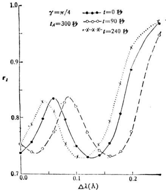
图 4 在阿尔文波波动周期内 I 轮廓的变化
