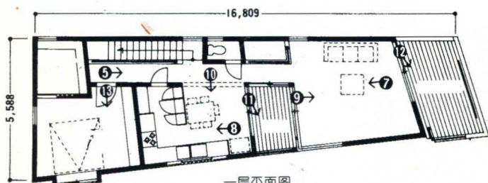
一层平面图
