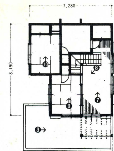
二层平面图
