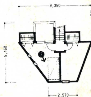
三层平面图
