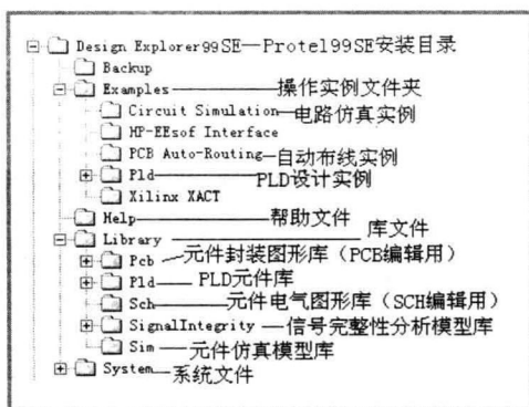
图 1-1 Protel 99 SE 安装后的文件结构
