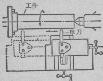
图 2-3 車床刀架的平动
