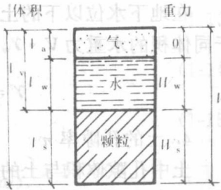
图 1-6 土的三相简图
