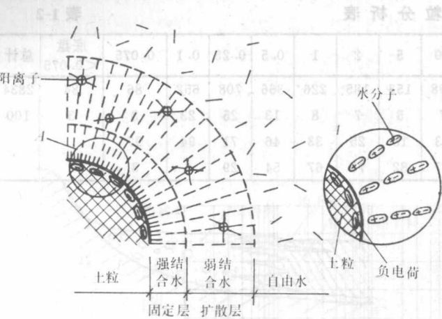
图 1-3 土中水的形态
