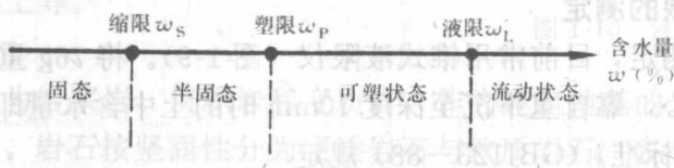
图 1-8 土的物理状态与含水量的关系
