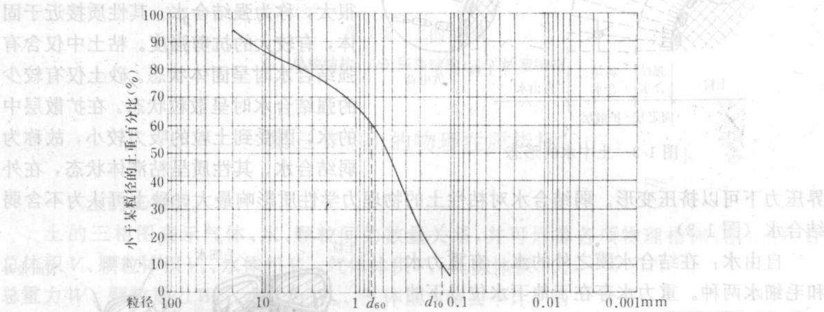
图 1-2 颗粒级配曲线示意图
