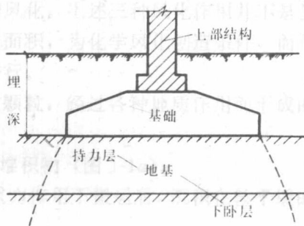
图 0-1 地基与基础示意
