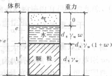
图 1-7 土的三相物理指标换算图
