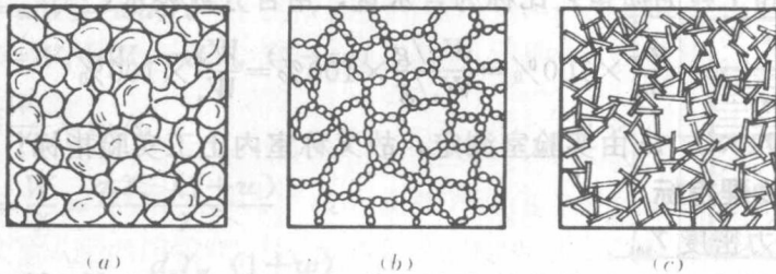
图 1-5. 土的结构
