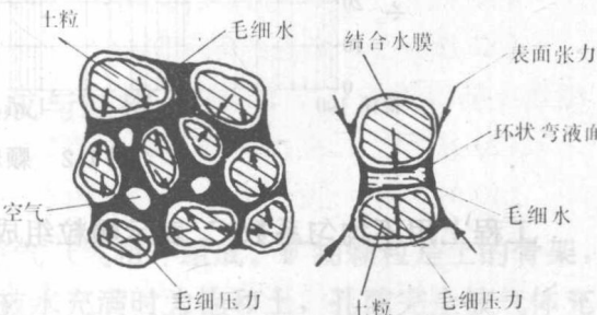
图 1-4 土粒间毛细水及毛细压力
