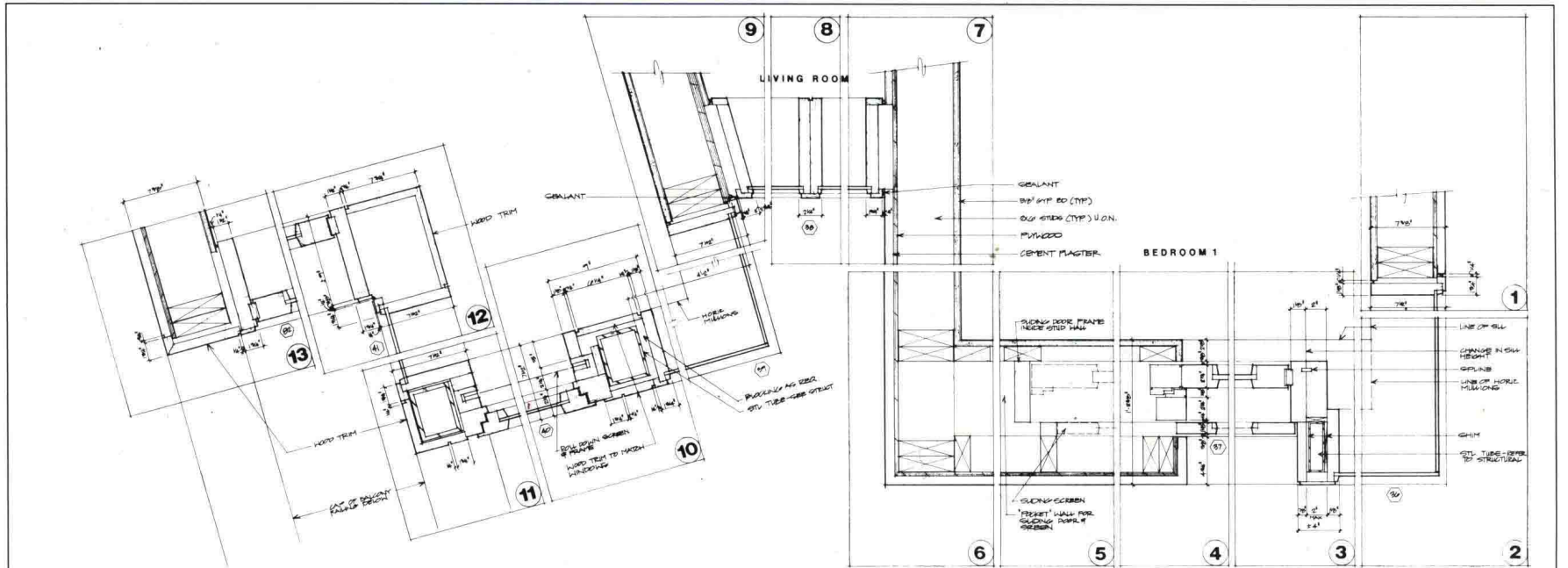
放大平面分解图 A. 主人卧室、起居室、卧室 I
