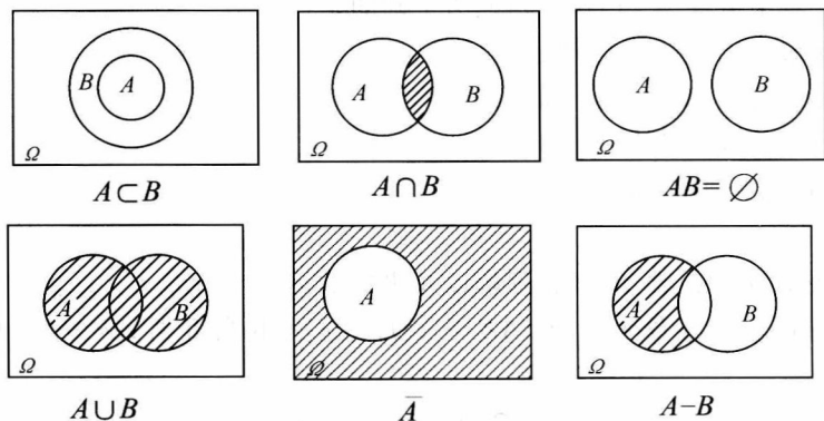
图 1-1 事件之间的关系与运算
