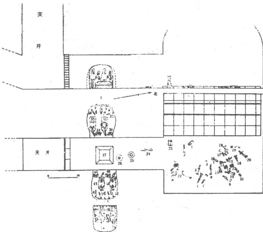
图二 墓葬平、剖面图
