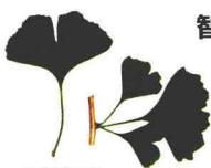
银杏叶
