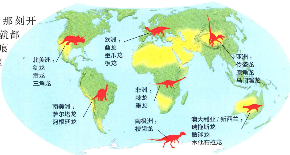
禽龙
