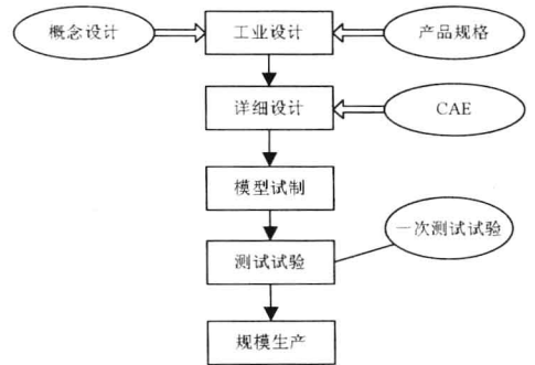
图 1-2 引入 CAE 后产品设计流程图
