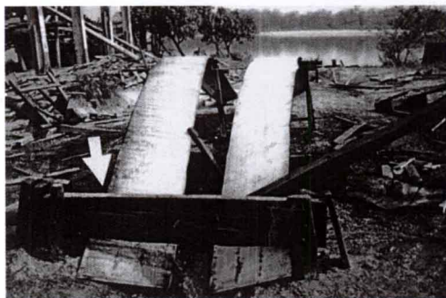
图四 上：木料加工场地“弯木地牛”遗迹
