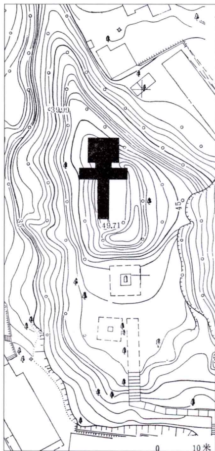
图五 南越文王墓位置示意图
