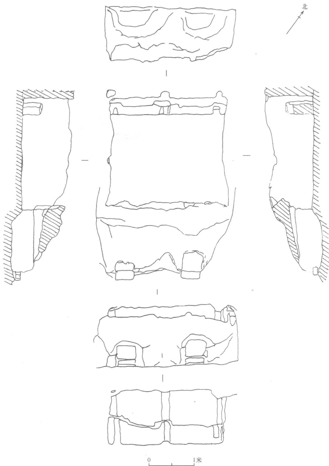
图一 余家嘴遗址陶窑 (Y1) 平、剖面图
