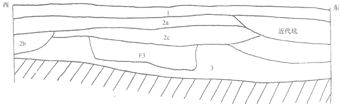
图八 T1、T2 北壁地层剖面图
