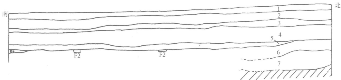
图七 T21B、T22B、T23B 西壁地层剖面示意图
