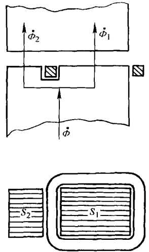
图 1-5 交流电磁机构短路环
