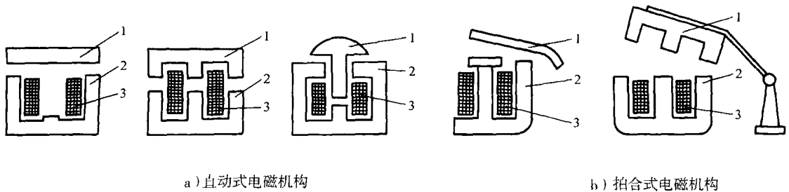
图 1-1 电磁机构
