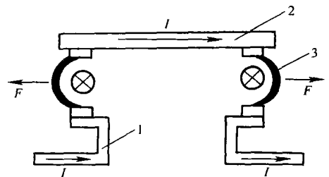
图 1-9 双断口电动力吹弧
