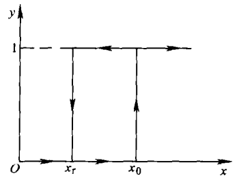
图 1-6 电磁机构的继电特性
