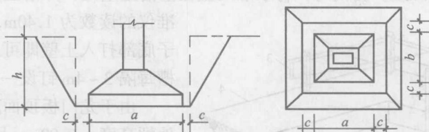
图 1-4 基坑土方量计算
