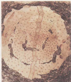
北魏 星象图 (1974年发现于河南洛阳市郊)
