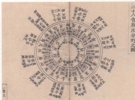
古代天文书籍中的二十八舍辰次分野图
