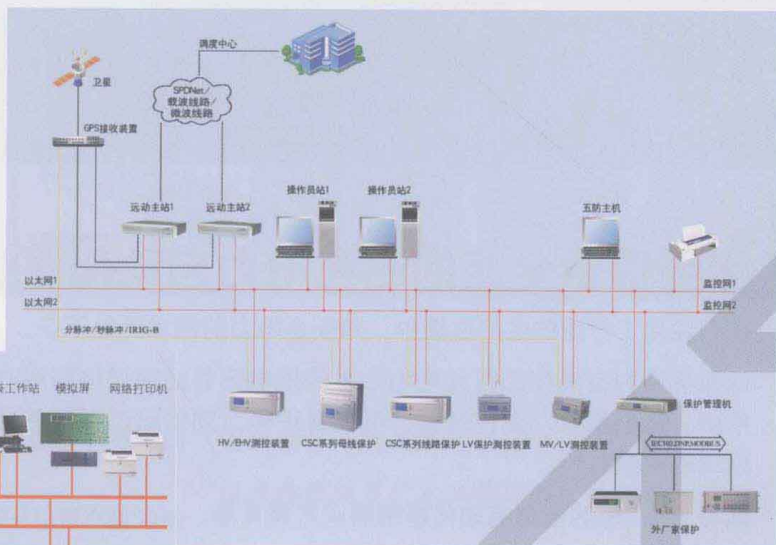
CSC-2000 (V2) 综自系统典型配置网络图
