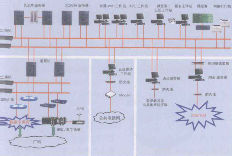
GC-3000集控站系统典型配置网络图
