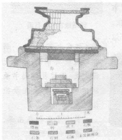
铁塔地宫结构图
