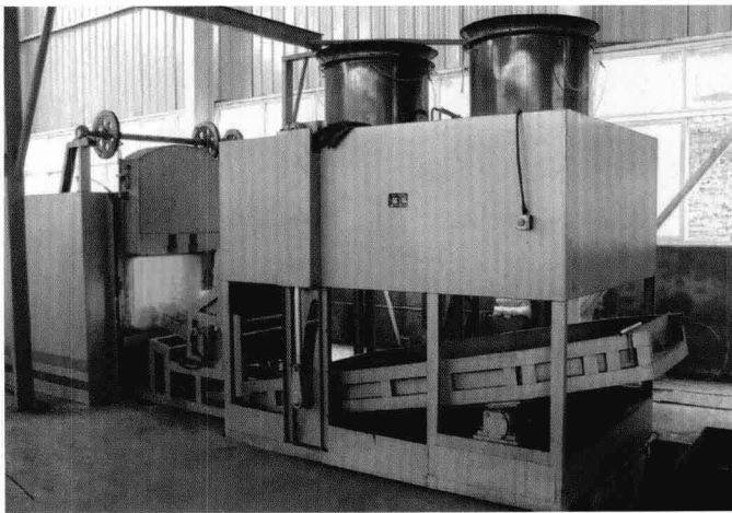
全自动推杆式淬火炉
