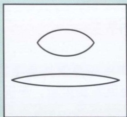
[ɔi]
