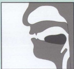
[ɔ:]
