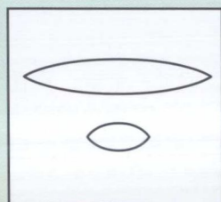
[əu]
