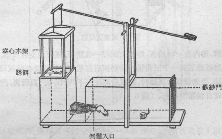
圖 4 木匣升降連續捕鼠箱
