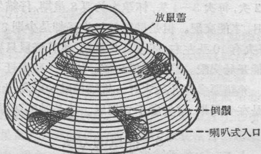
圖 2 倒鬚捕鼠籠
