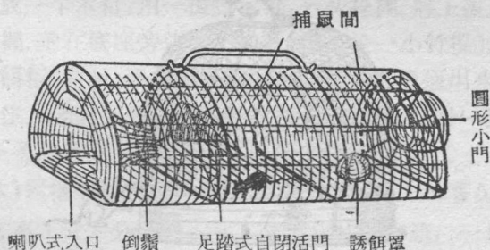
圖1 印度式捕鼠籠
