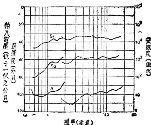
圖 19.1 靈敏度特性曲線
