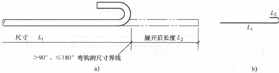
图 1-15 大于 90°、不大于 180°弯钩的标注
