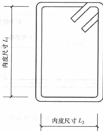
图 1-17 内皮尺寸
