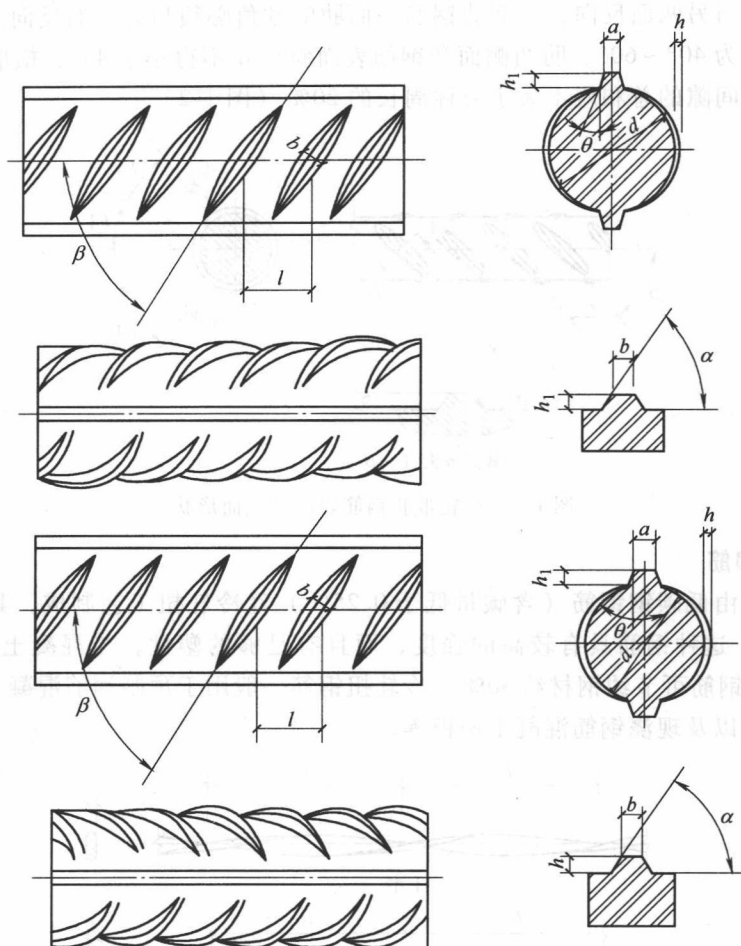
图 1-1 月牙肋钢筋（带纵肋）表面及截面形状
