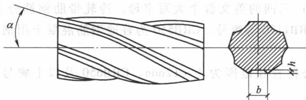
图 1-4 冷拔螺旋钢筋表面及截面形状
