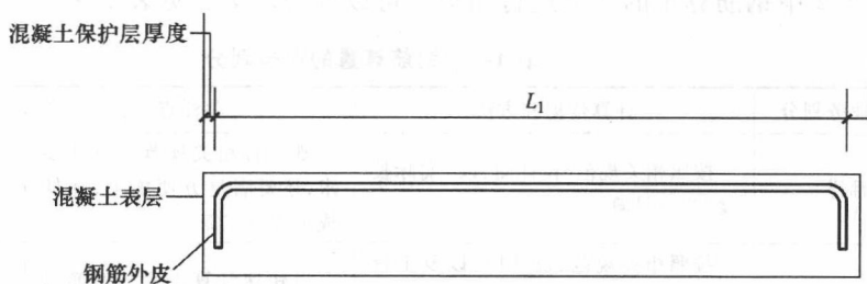
图 1-9 设计尺寸
