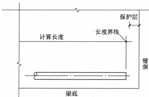
图 1-13 直形钢筋计算长度
