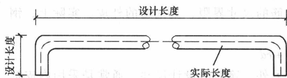
图 1-6 实际长度
