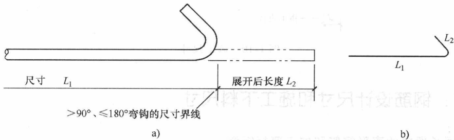
图 1-16 拉筋尺寸标注
