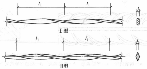
图 1-3 冷轧扭钢筋表面及截面形状
