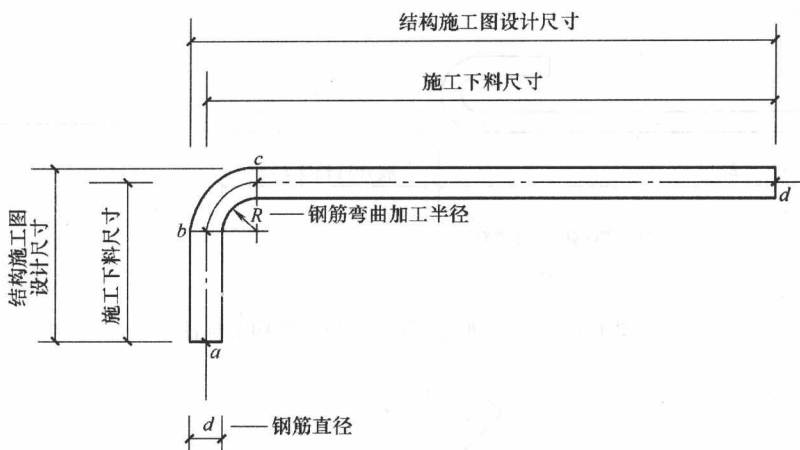
图 1-10 施工尺寸
