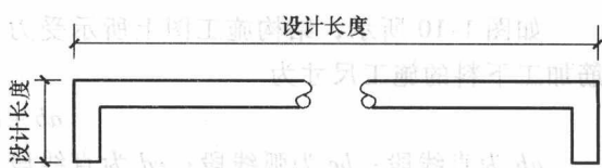
图 1-7 设计长度
