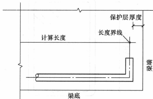
图 1-14 弯折钢筋计算长度
