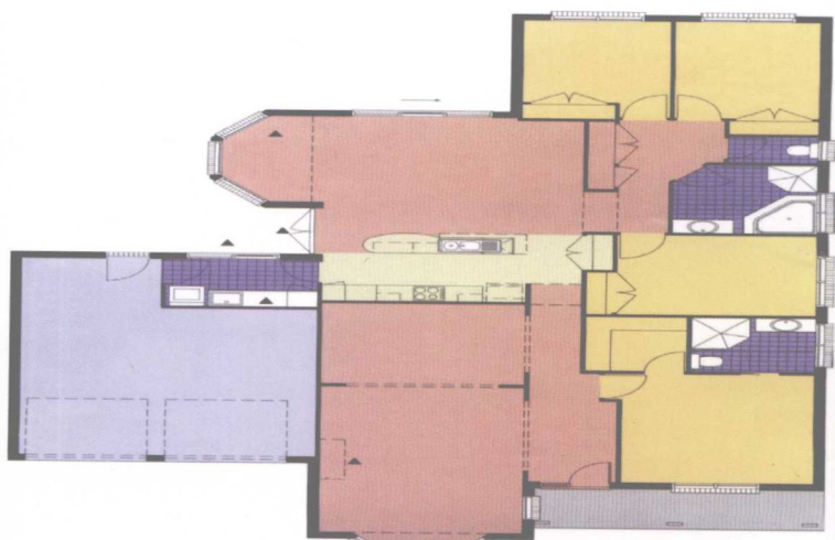
首层平面图
