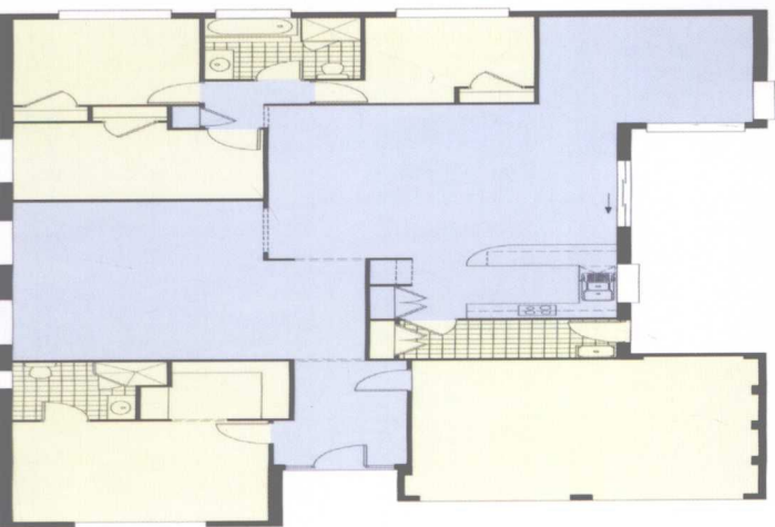
首层平面图
