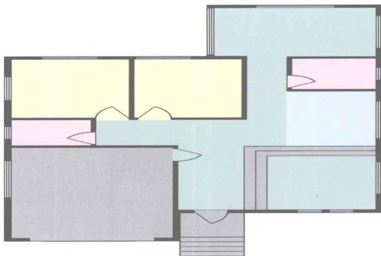
首层平面图
