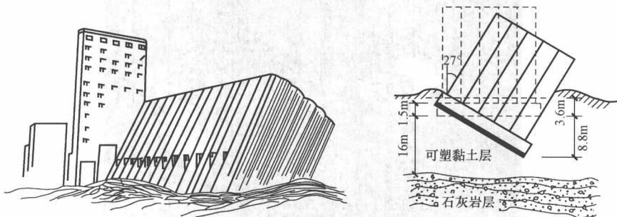
图 1-4 加拿大特朗斯康谷仓
