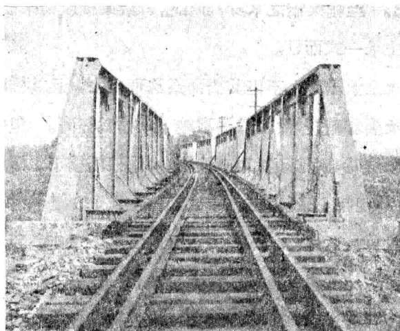
影片 X. 矮桁架橋(軌道係曲線)
