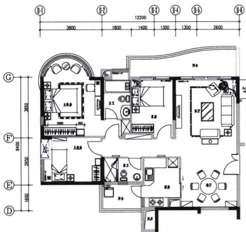
平面布置图
