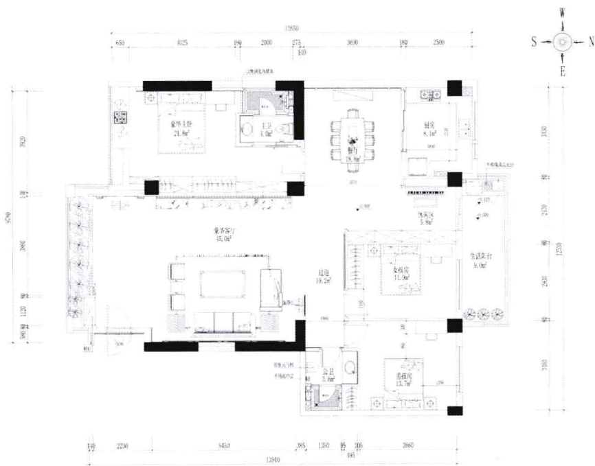
平面布置图
