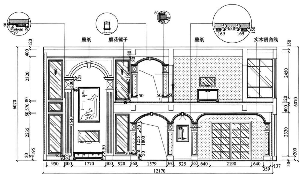
客餐厅A立面图
