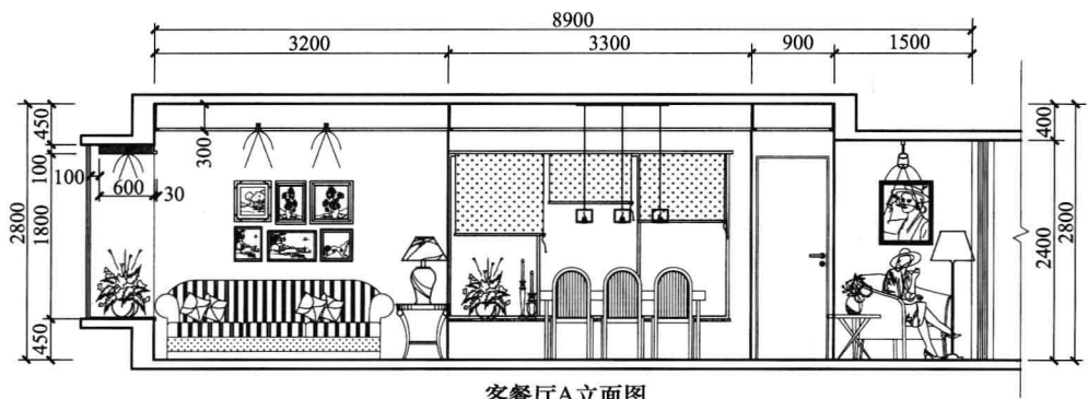
客餐厅A立面图
