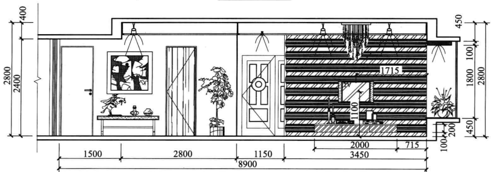
客餐厅B立面图
