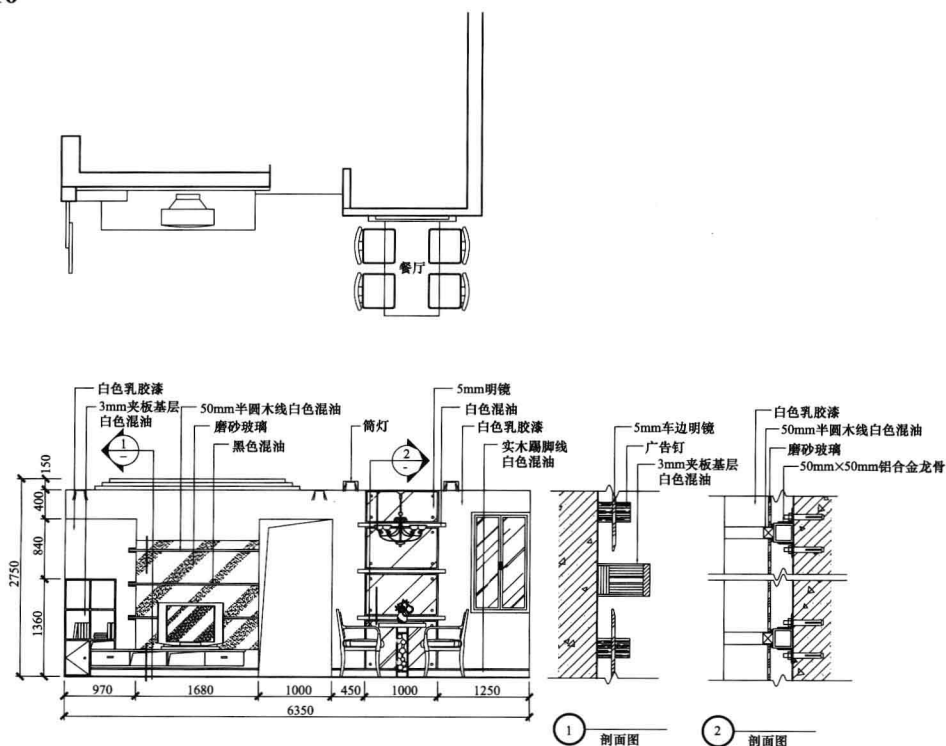
客餐厅电视墙立面图
