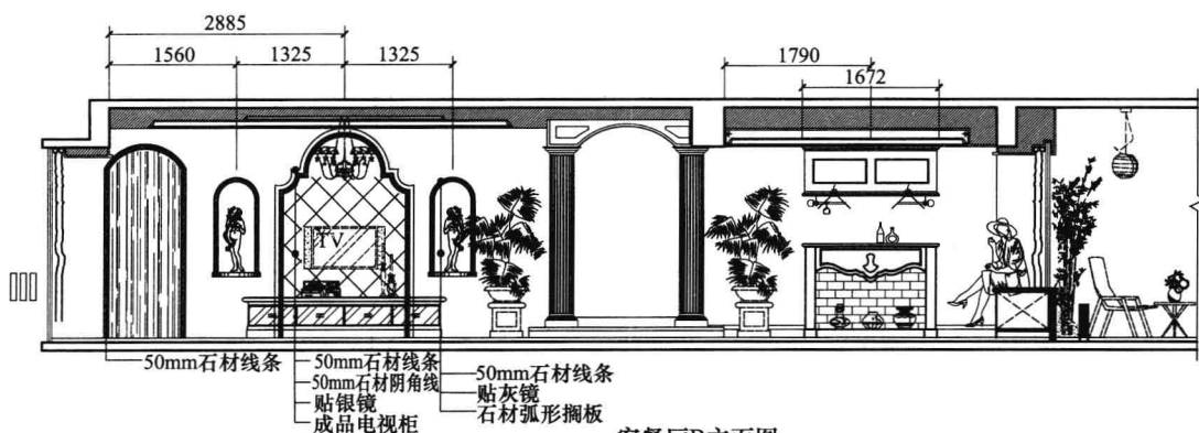
客餐厅B立面图
