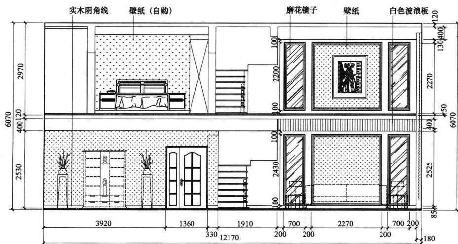
客餐厅B立面图
