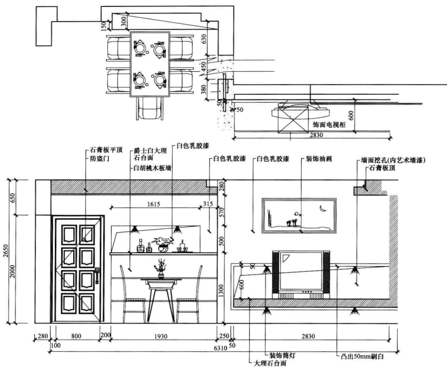
客餐厅电视墙立面图
