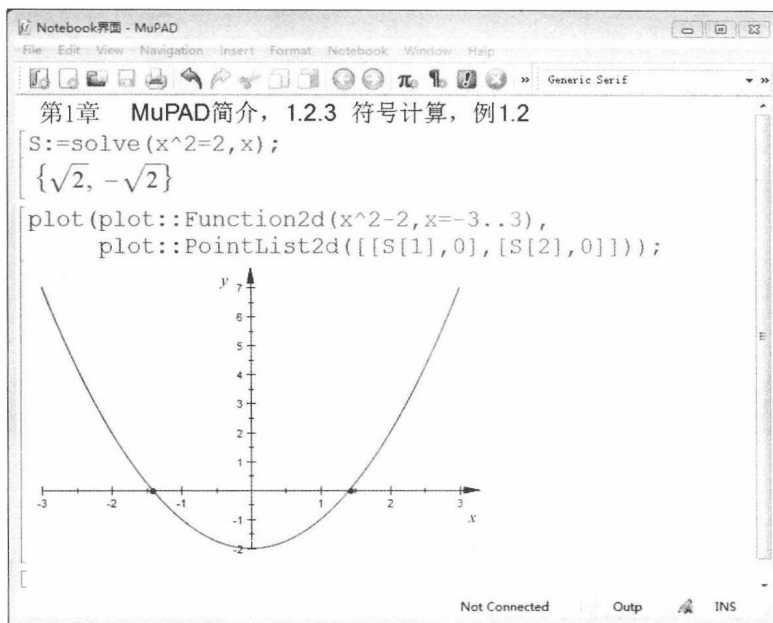
图 1.2 Notebook 界面
