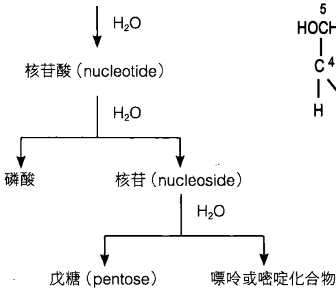
核糖 (ribose)
