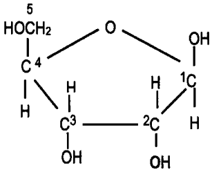
核糖 (ribose)
