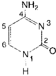
嘧啶 (pyrimidine)
