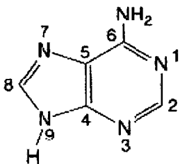
嘌呤 (purine)
