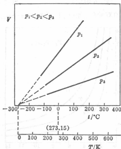
图 1-3 理想气体的 V - T 图
