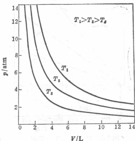
图 1-1 理想气体的 p - V 图
