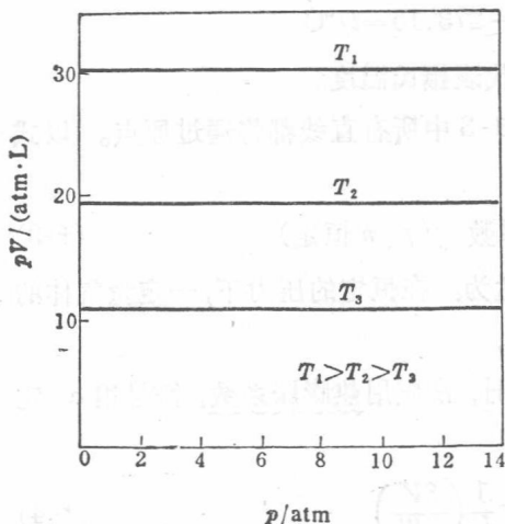
图 1-2 理想气体的 pV - p 图
