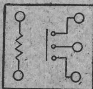
图1-3 JC-21型内部接綫
