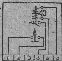
图 1-16 RZf型接线
