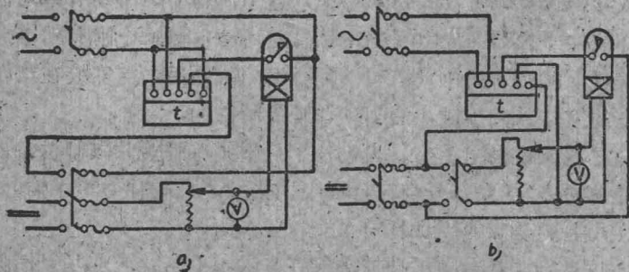
图 1-11 延时复归中間繼电器时间特性試驗
