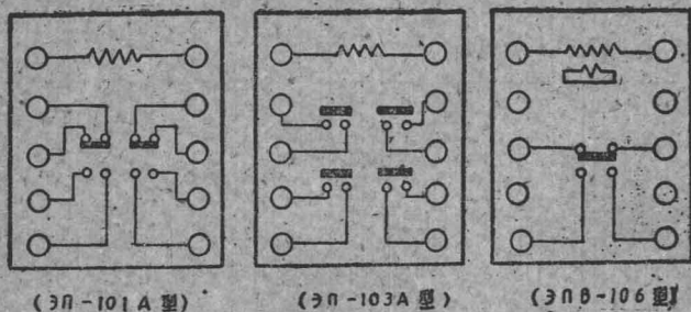
图 1-5 ЭП-100型中间继电器接线
