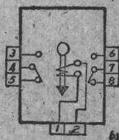
图1-4 RA型信号繼电器接綫
