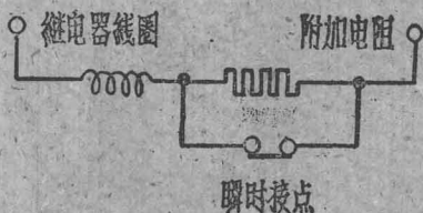
图 1-13 9B型時間繼電器長時間通电接綫方法
