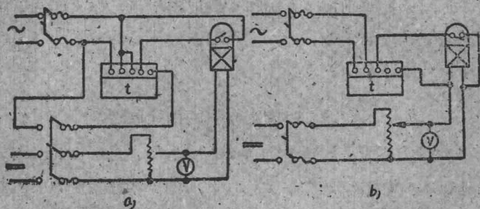
图 1-10 中間繼电器动作时间試驗接綫
