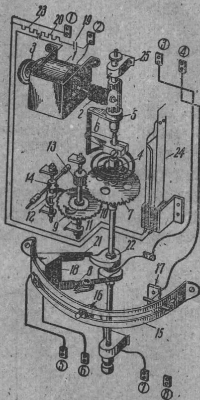
图 1-12 JB-180型时间继电器的构造
