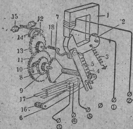
图 1-14 PB型時間繼電器的構造
