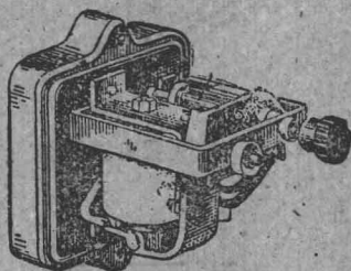
图 1-1 信号继电器构造
