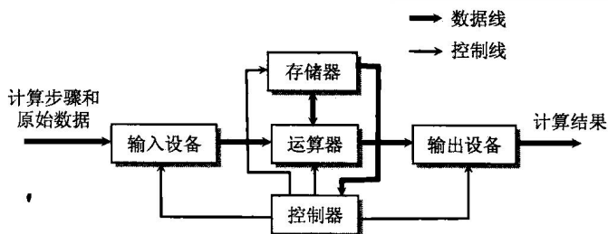
图 1.1 典型的冯·诺依曼计算机结构图
