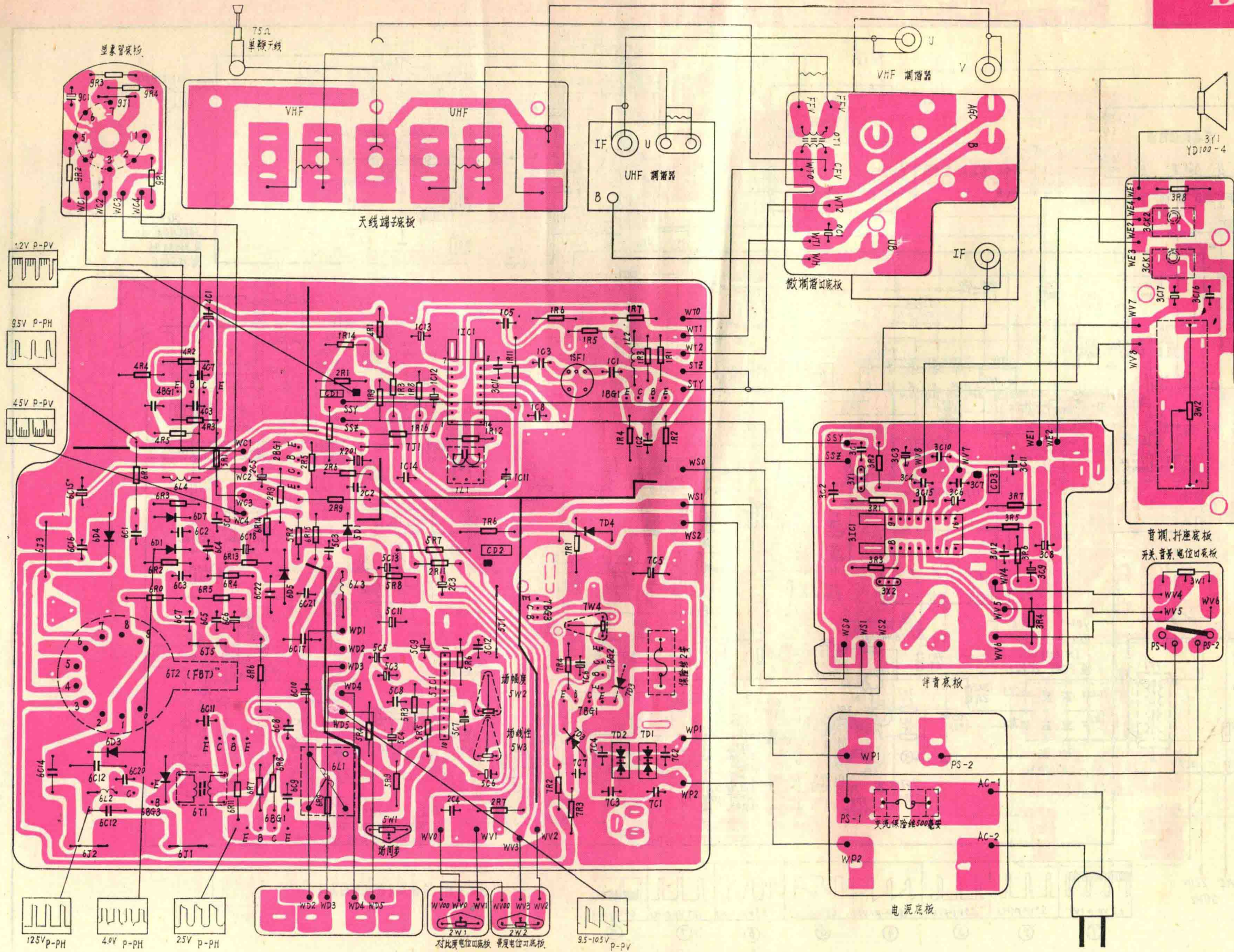
印制板图
