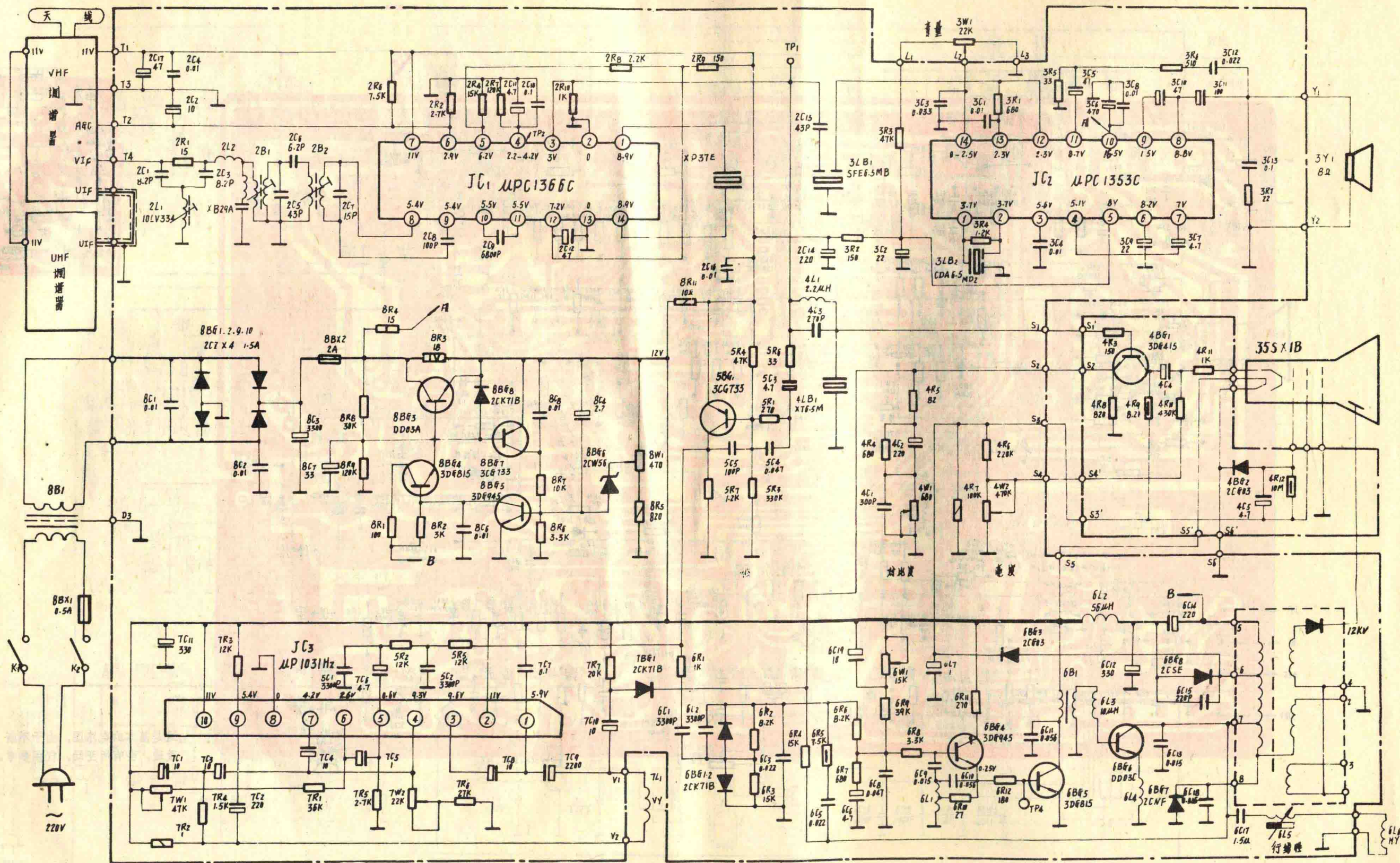
电原理图
