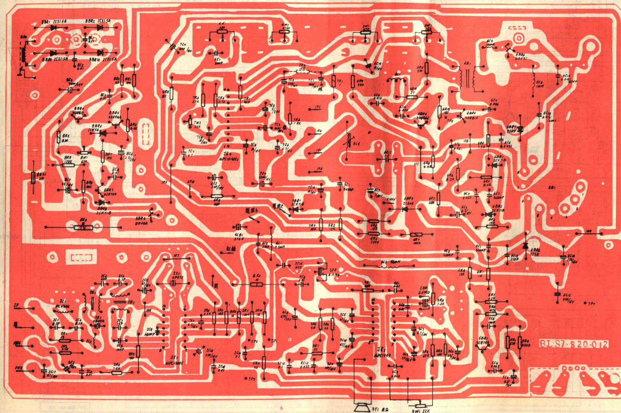
印制板图
