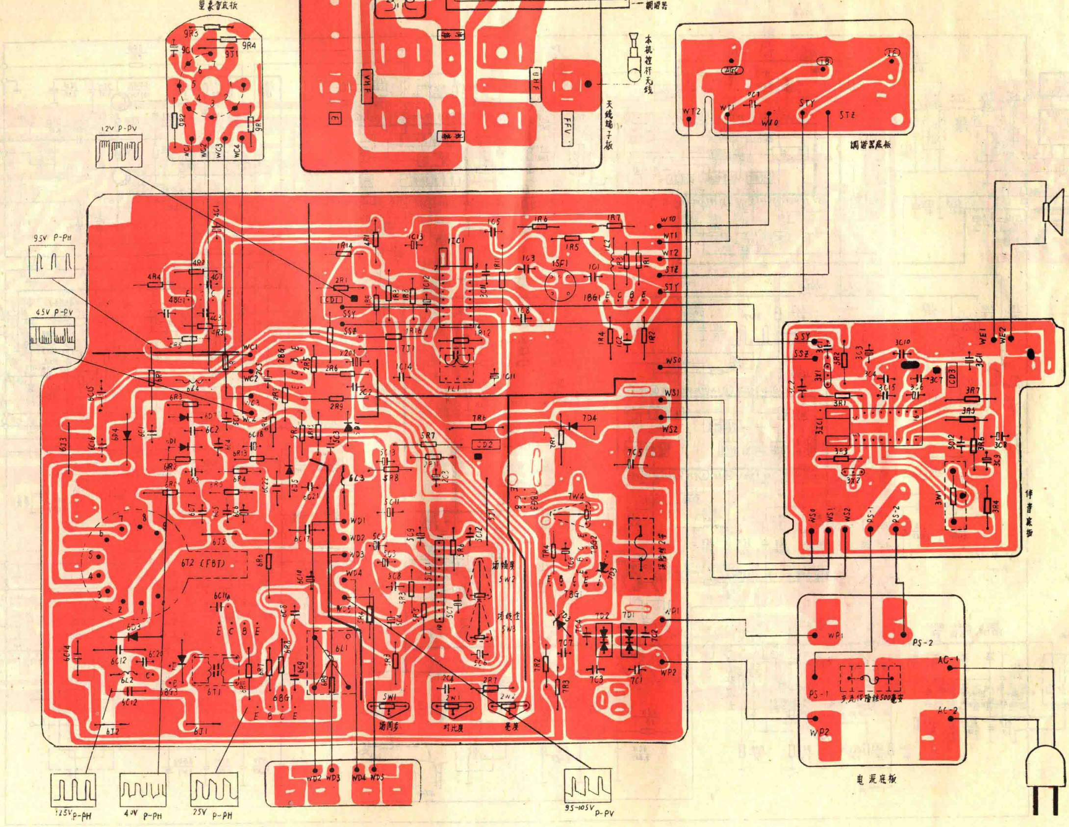
印制板图
