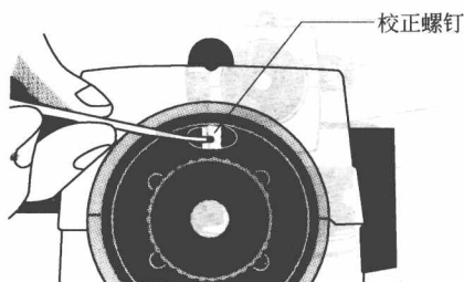
图 4-5 调整分划板校正螺钉
