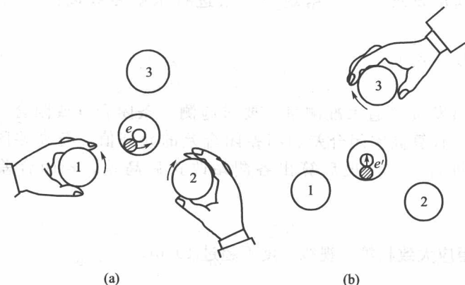
图 1-1 概略整平方法
