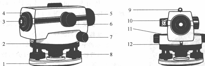
图 4-1 DS32 自动安平水准仪的外部结构
