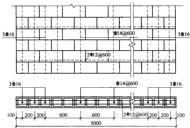
图 1.1.5 配筋砌块砌体剪力墙
