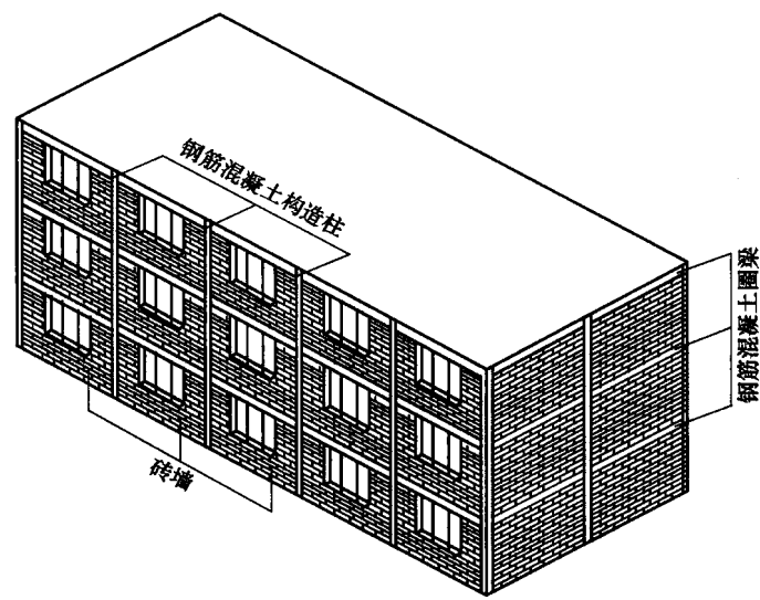
图 1.1.4 内嵌式组合砖墙
