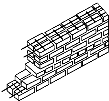
图 1.1.2 水平配筋砖墙
