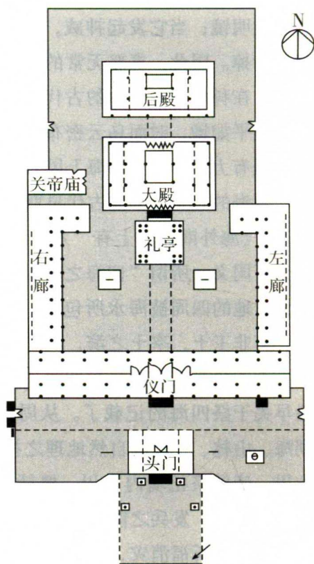
南海神庙平面图
