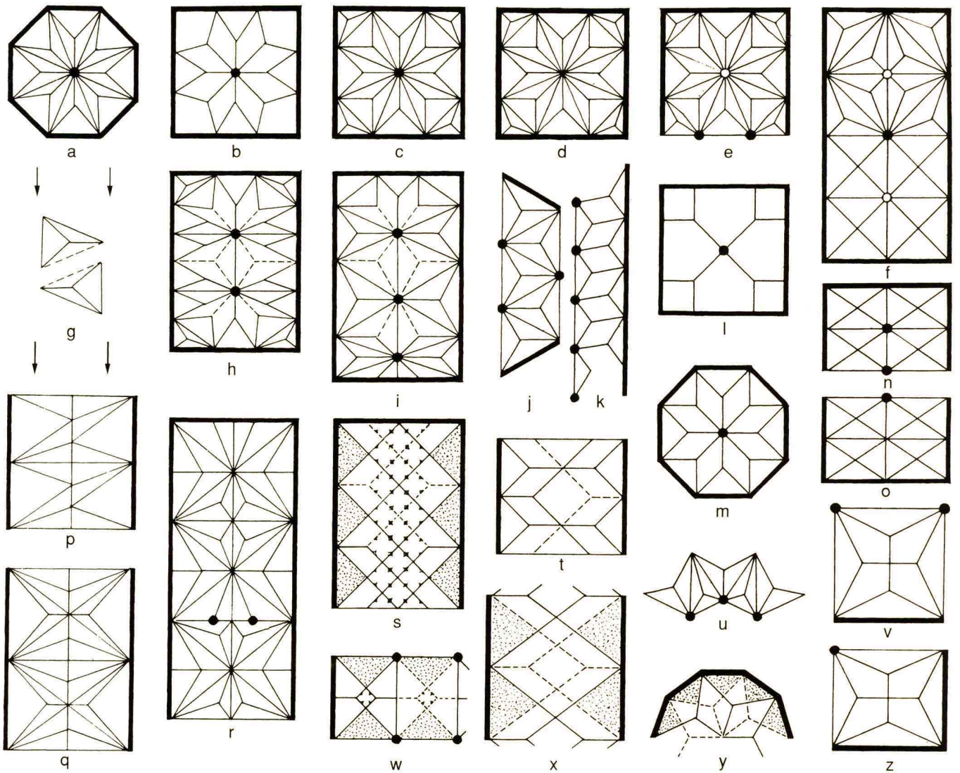
图5-1 中欧及英国哥特拱顶平面略图 (未按统一比例; 黑圆圈为柱墩, 空心圆圈示垂饰, 虚线表示大尺度的三射线, 打点区标出筒拱的切入部分)。图中: a、以伦敦西寺为代表的英国教会堂; b、维拉尔·德奥纳库尔图样所示教会堂方案; c、埃伯巴赫教会堂; d、布尔戈斯大教堂教会堂; e、斯特拉斯堡大教堂圣凯瑟琳礼拜堂跨间之一; f、布拉格大教堂圣器室; g、双三射线拱顶; h、吕贝克圣母院圣安娜礼拜堂; i、毛尔布龙教会堂; j、布拉格大教堂南耳堂门廊拱顶; k、兹维科夫城堡柱廊院; l、上布罗德教会堂; m、库里姆圣司提反教堂地下室; n、林肯大教堂本堂北侧礼拜堂; o、林肯大教堂本堂南侧礼拜堂; p、林肯大教堂歌坛主跨; q、林肯大教堂本堂主跨; r、伦敦西寺官殿圣司提反礼拜堂底层, 后殿及本堂一跨间; s、奥特里圣玛丽圣母礼拜堂; t、布拉格查理桥老城塔楼入口厅; u、科林回廊部分; v、兰茨胡特圣马丁教堂本堂边廊; w、奥特里圣玛丽圣母礼拜堂屏栏 (三跨中的两跨); x、布拉格大教堂歌坛中央空间; y、布拉格大教堂歌坛半圆室; z、斯海尔托亨博斯南耳堂门廊 (三跨中的一跨)
