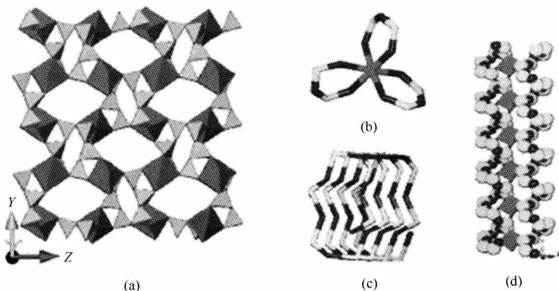
图 1-2 (a) TbSiO-CJ1 沿 [100] 方向的三维骨架结构; (b) 螺旋桨构型的手性结构单元 [TbSi_6 O_9] ; (c) 沿 [100] 方向 2_1 螺旋轴无限延伸的左手螺旋链; (d) 相邻的螺旋链通过 TbO_6 连接构成 TbSiO-CJ1 三维骨架 [44]
