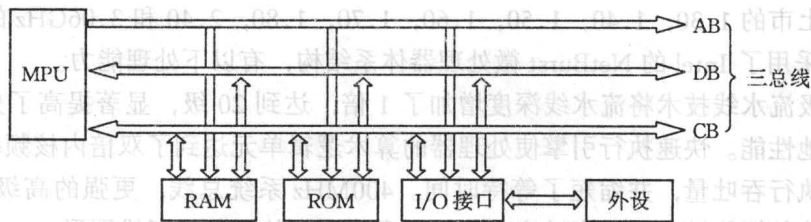
图 1-1 微型计算机结构框图
