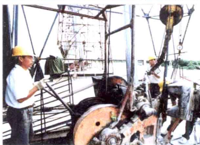
施工单位在向钻孔内注浆。(2003年8月12日)
