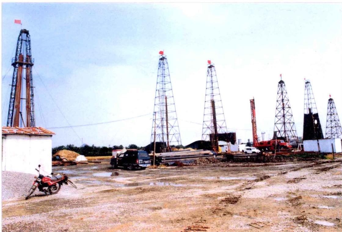
东庞矿“4·12”突水灾害抢险，打钻注浆堵水施工现场。
