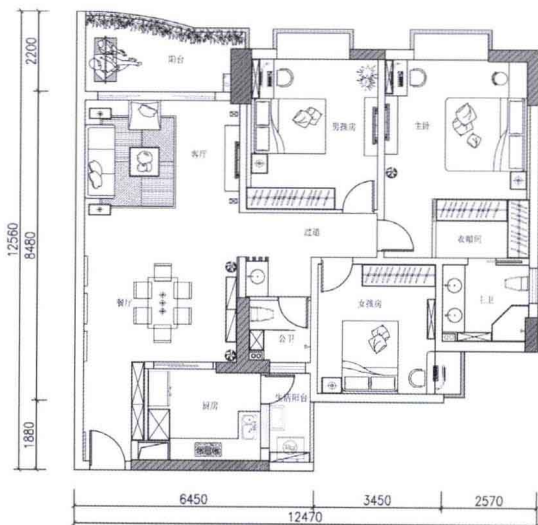
平面图
