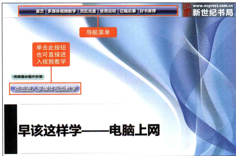
图1 光盘主界面
