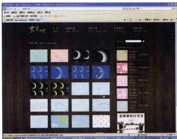
图3 全屏显示
