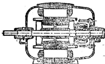
圖 1-6 直流電機
