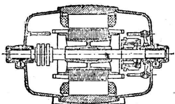
圖 1-16 單樞換流機
