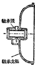
圖 1-4 拖動端的軸承端蓋
