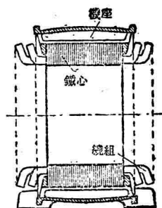
圖 1-3 定子的組成部分
