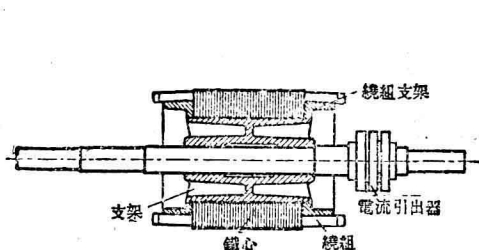
圖 1-2 轉子的組成部分
