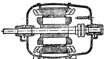
圖 1-12 同步電機
