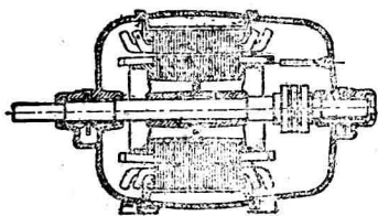
圖 1-8 滑環式感應電動機
