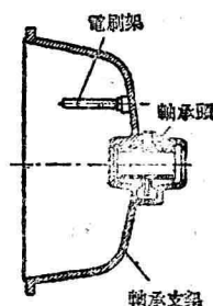
圖 1-5 電刷端的軸承端蓋
