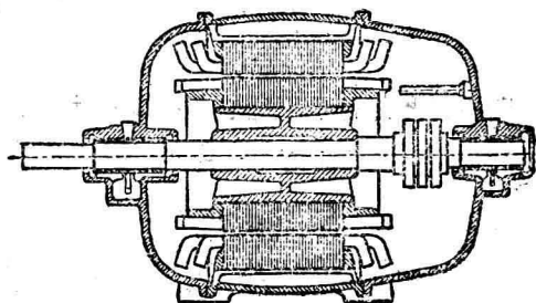
圖 1-1 感應電動機（一覽圖）
