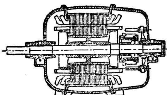
圖 1-14 交流電整流子電機
