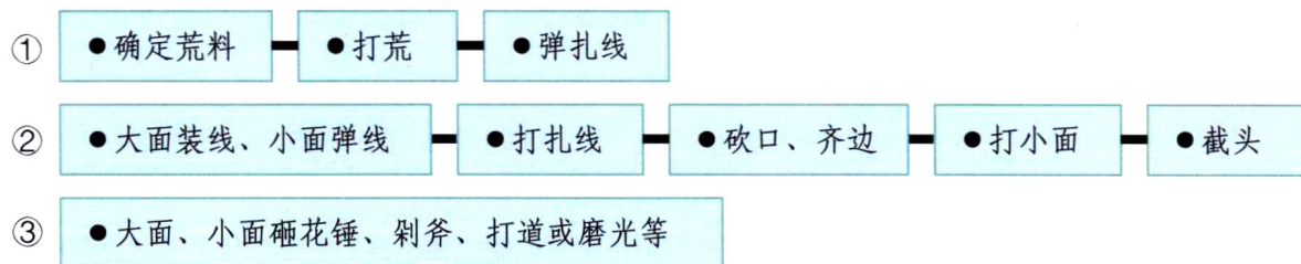
图1-10 石料加工的基本工序图
