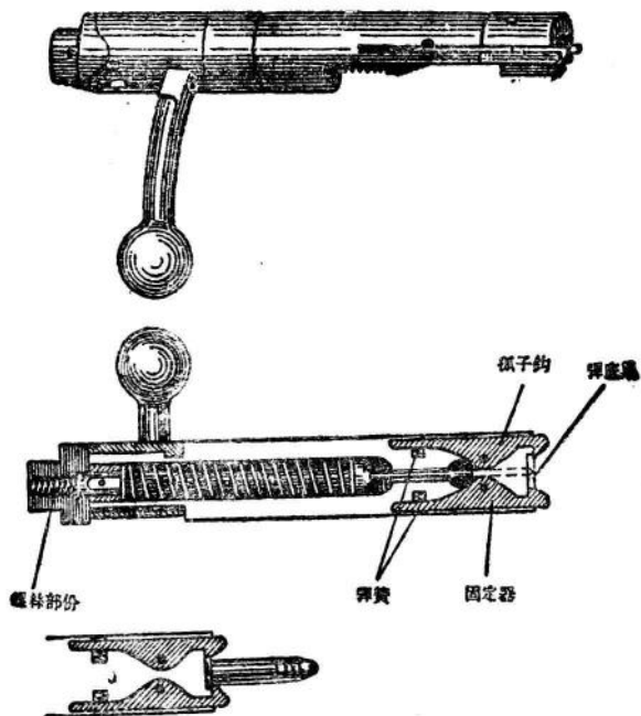
圖五：槍機
