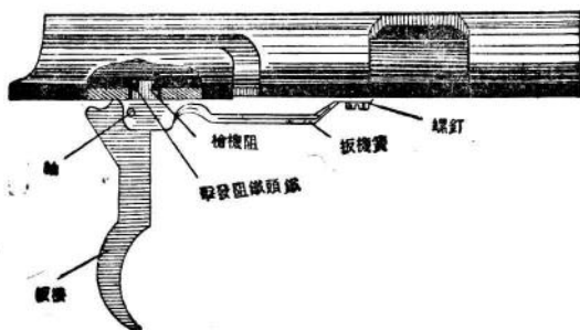
圖六：擊發機
