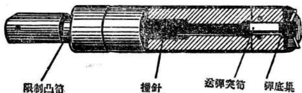
圖九：機體
